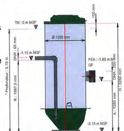
Schéma du poste de refoulement
